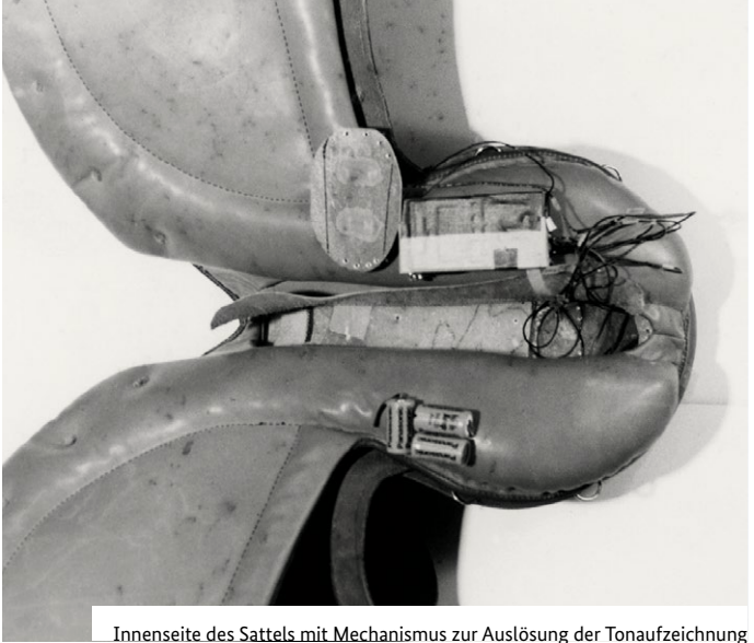
Innenseite des Sattels mit Mechanismus zur Auslösung der Tonaufzeichnung
